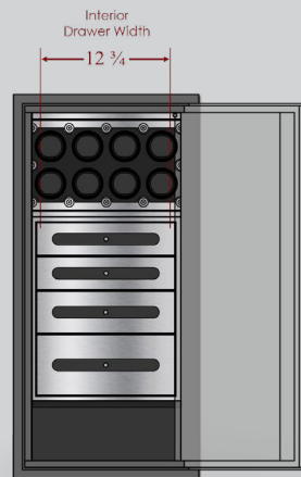
135° Door Swing
